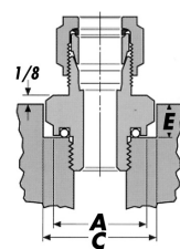
Montage dans lamage profond
