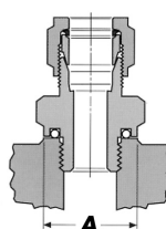
Montage sur bossage
