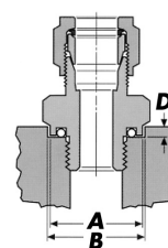
Montage dans lamage court
